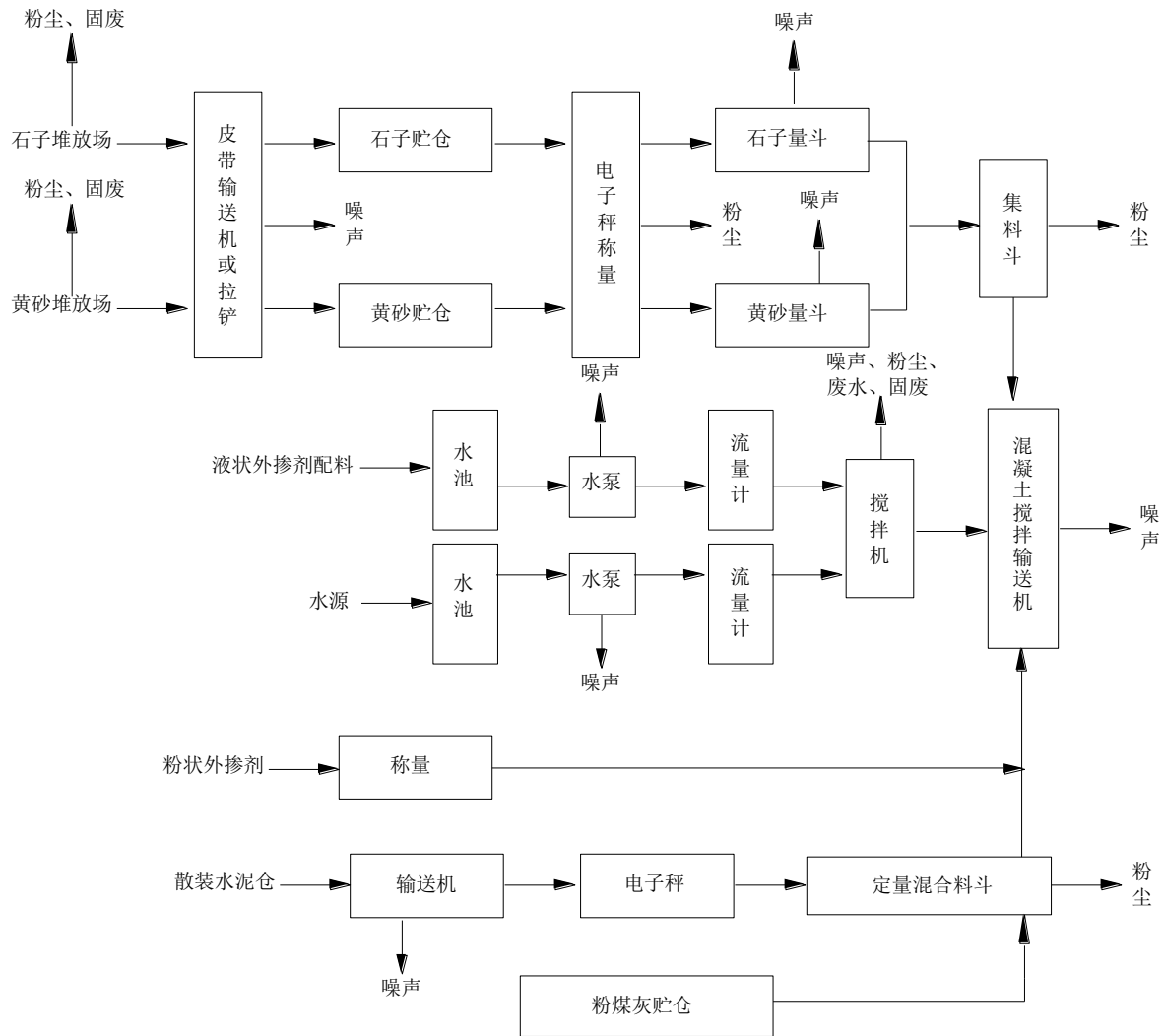
图 3-4 商品混凝土生产工艺及产污流程
