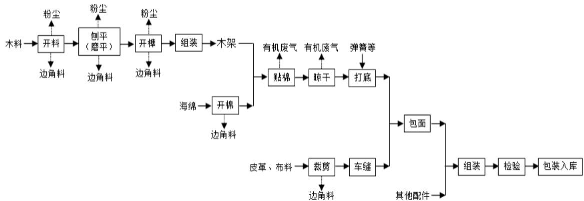
图3-2 生产工艺流程图
