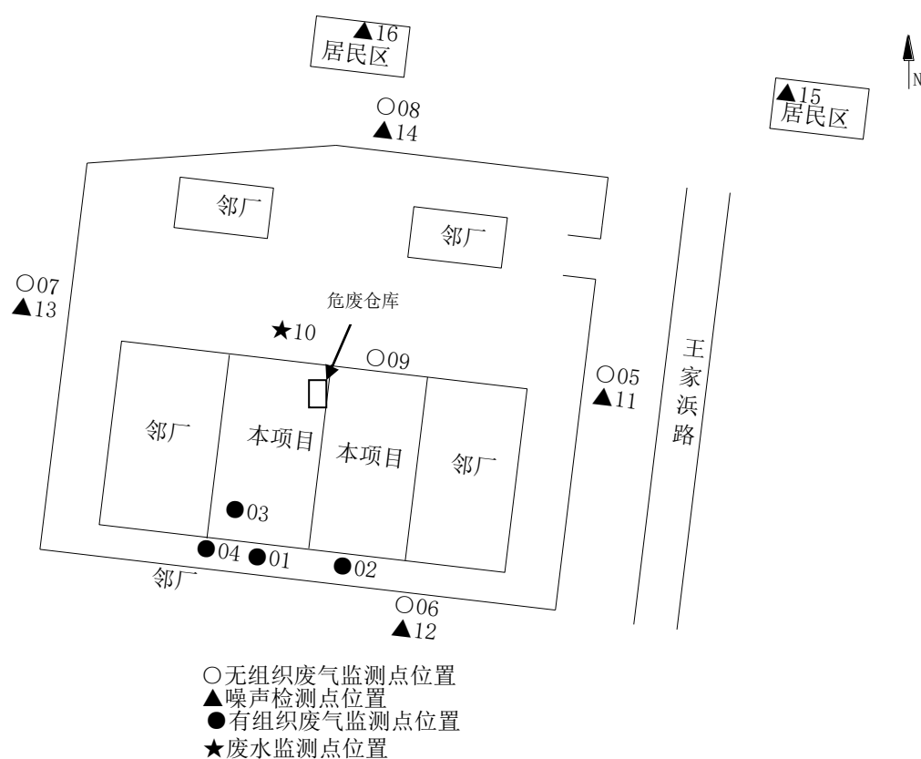
图 3-2 项目厂区总平面布置图
