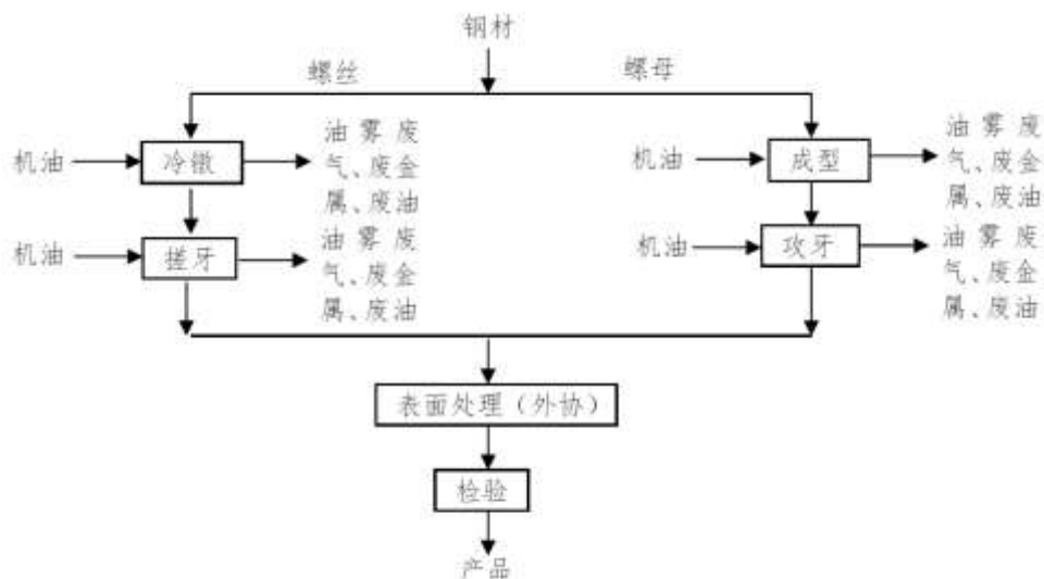
图 3-4 本项目高强度紧固件生产工艺及产污流程图
