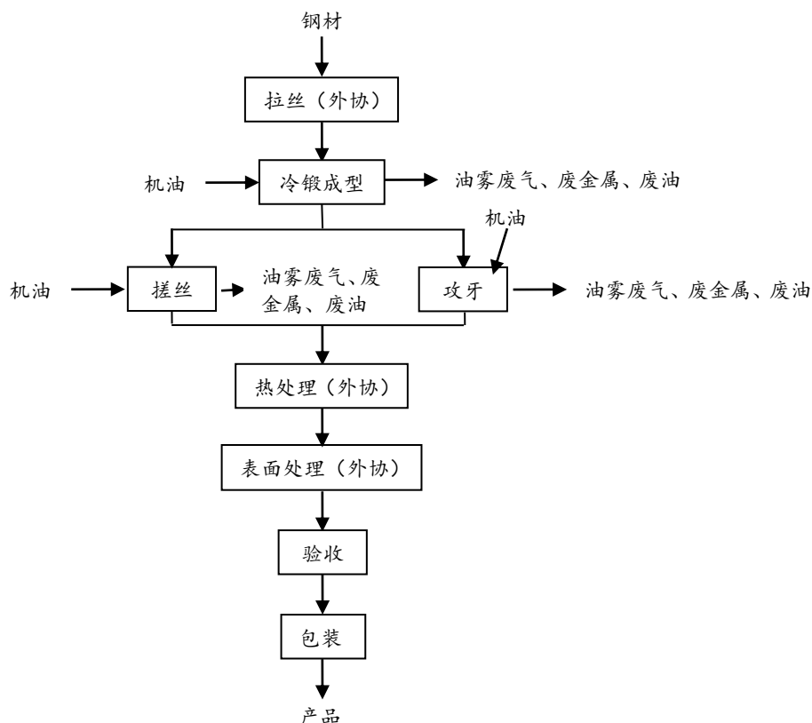
图 3-4 本项目生产工艺及产污流程图
