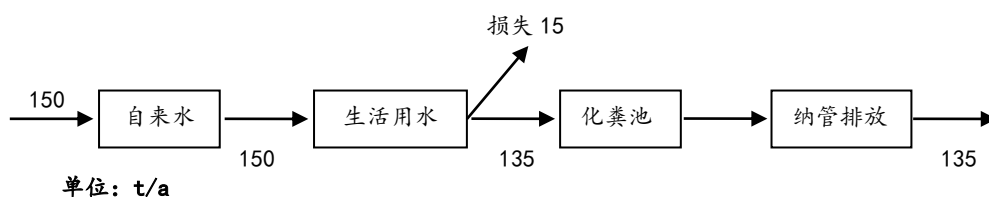
图 3-3 水量平衡图
